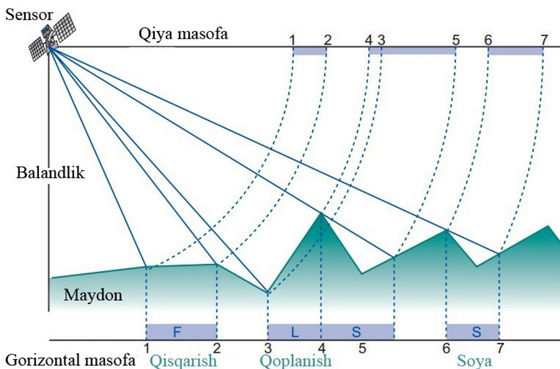
4.6-rasm. Maydon balandligi tufayli radar tasvirda geometrik buzilishlar(Manba: 6 adabiyot).
