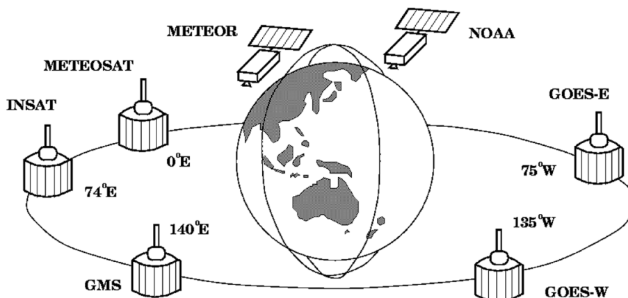
3.13-rasm. Geostatsionar va qutbiy sun‘iy yo‘ldoshlardan tashkil topgan meteorologik kuzatish tizimi (Manba: 6 adabiyot).
