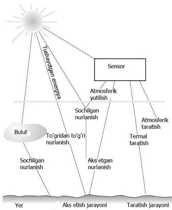
2.8-rasm. Atmosferada va Yerdagi energiyaga ta'sirlar (Manba: 6 adabiyot).
