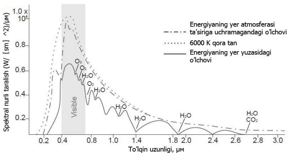
2.13-rasm. Quyoshning elektromagnit spektrni Yer atmosferasi ta'siri bo'lgan va bo'lmagan holatlaridagi kuzatishlar (Manba 6 adabiyot).
