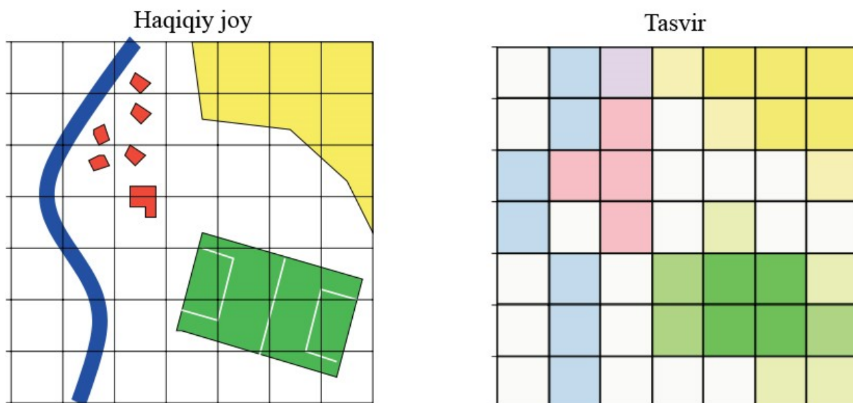
7.15-rasm. Aralash piksellar: turli yer qoplami turlari bitta pikselga tushadi.
