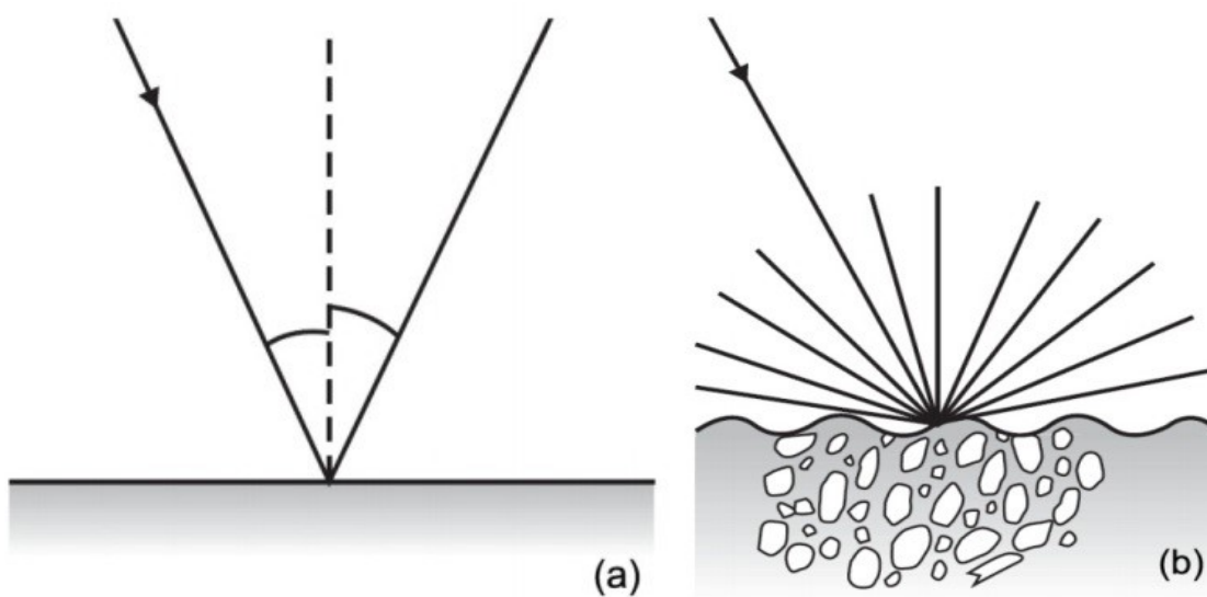
2.14-rasm. (a) ko'zguli va (b) tarqoq qaytishning sxematik diagrammasi (Manba: 6 adabiyot).
