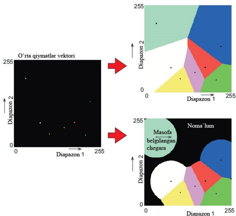
7.13-rasm. Ikki o'lchamli holatda minimum masofali sinflash tamoyili. Yechim chegaralari chegaraviy masofasiz (yuqoridagi o'ng) va chegaraviy masofa (pastgi o'ng) holatlarida keltirilgan (Manba: 6 adabiyot).
