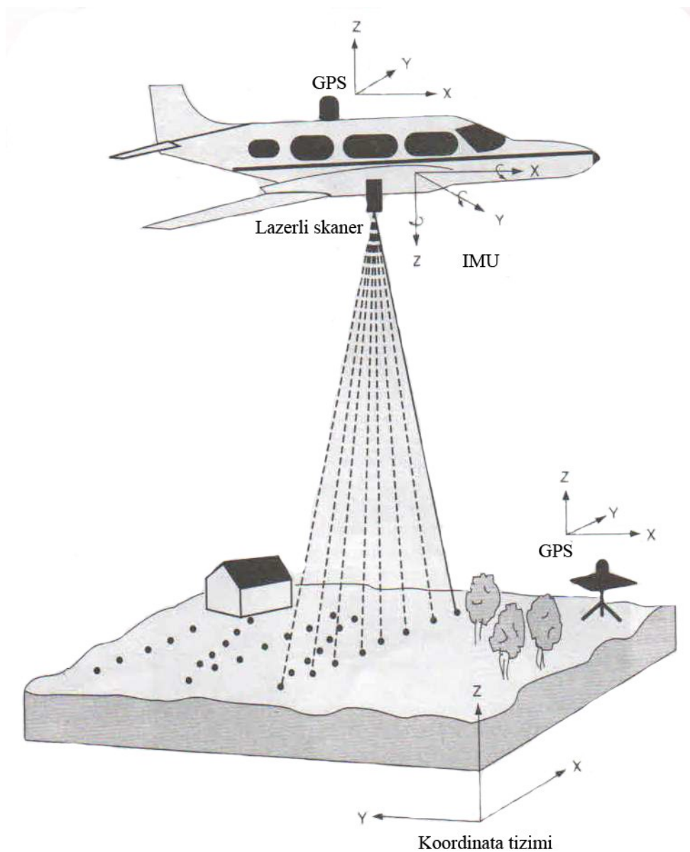
4.9-rasm. Havodan lidar skanerlash tizimining tarkibiy qismlari(Manba: 5 adabiyot).
