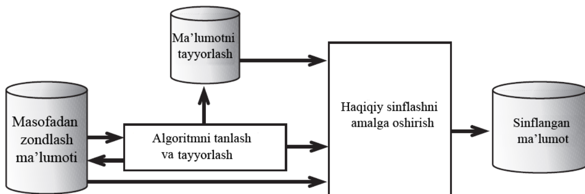
7.6-rasm. Sinflash jarayoni.
