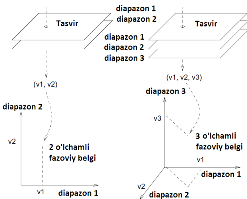
7.2-rasm. Fazoviy tekislikda ikki va uch diapazonli tasvir uchun piksel qiymatlarini grafik tasvirlash (Manba: 6 adabiyot).
