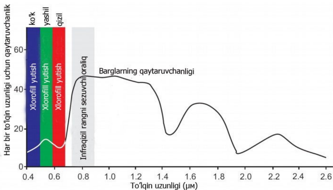
2.15-rasm. Sog‘lom o‘simlikning qaytarish egri chizig‘I (Manba: 6 adabiyot).
