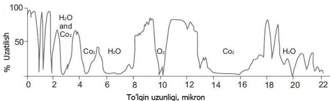
2.12-rasm. Atmosferik uzatilish foizlarda keltirilgan (Manba: 6 adabiyot).
