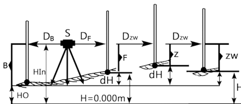
2.19-rasm. DNA raqamli nivelir bilan ishlash sxemasi:
