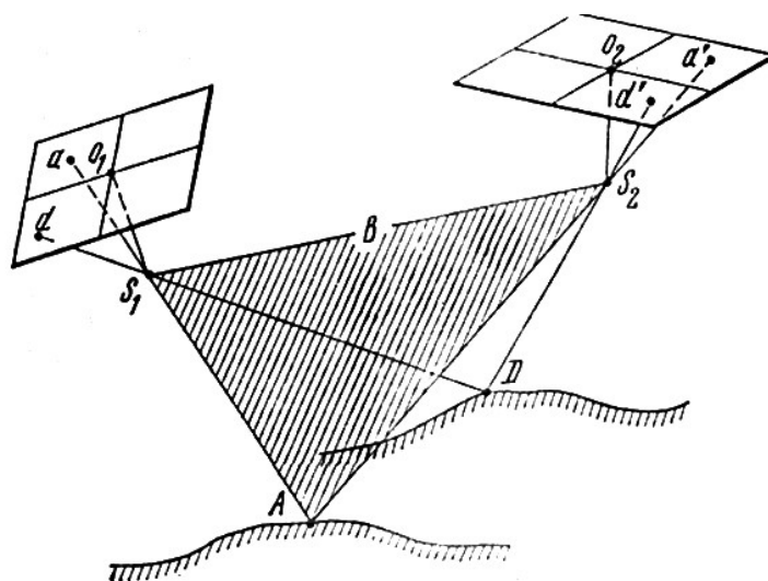
4.23-rasm. Fazoviy kesishtirish
