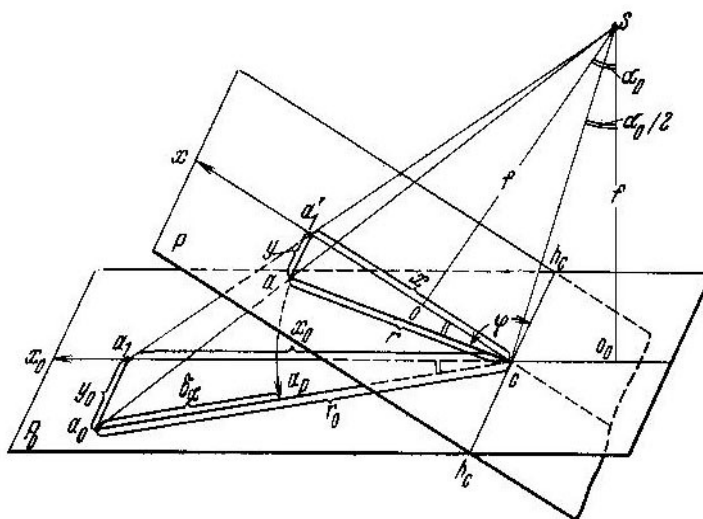
4.11-rasm. Gorizontol va og'ish burchagi bo'lgan aerofotosurat orqali chiziqli xatoliklarni aniqlash
