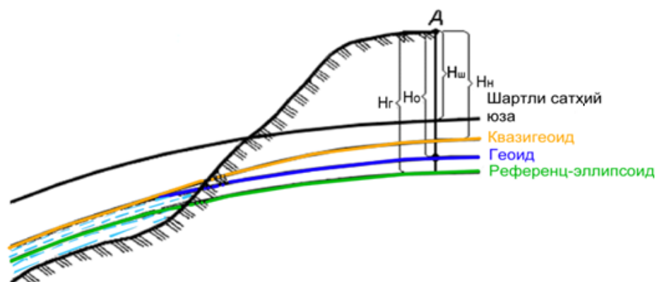
1.12-rasm. Geodeziyada balandliklar sistemasi
