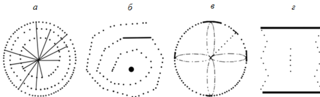
2.11-rasm. Elektron-blokli taxeometriyada piket nuqtalari s'yomkasining sxemalari:
