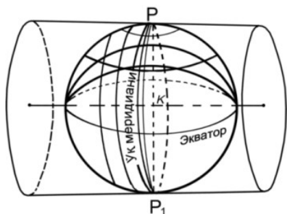
1.24-rasm. Gauss-Kryuger ko'ndalang-tsilindrik proektsiyasi
