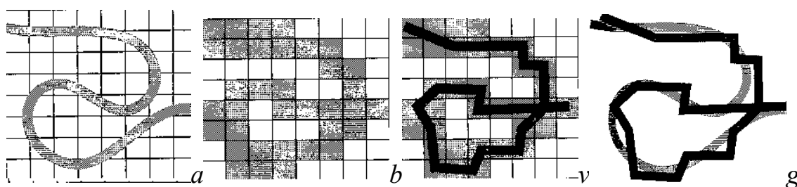
5.13- shakl. Rastr va vektor formatlardagi ma'lumotlar.
