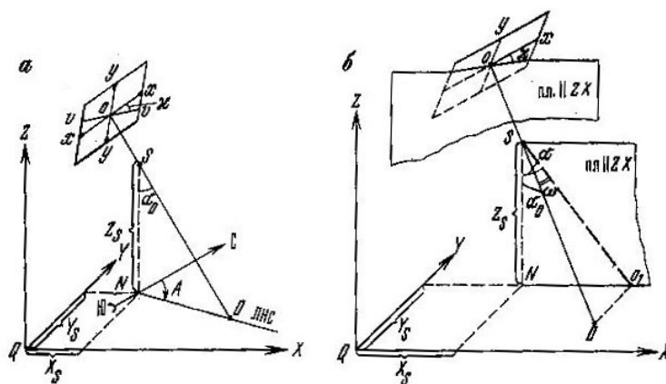
4.19-rasm. Tashqi orientirlash elementlari:
