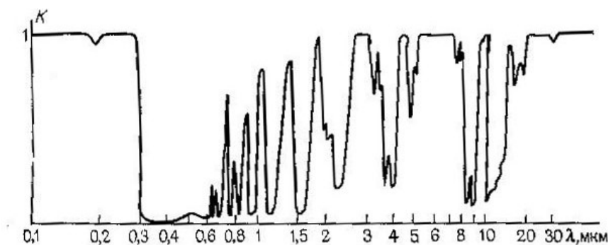
4.2-rasm. Atmosferaning to'lqinlarni yutish grafigi
