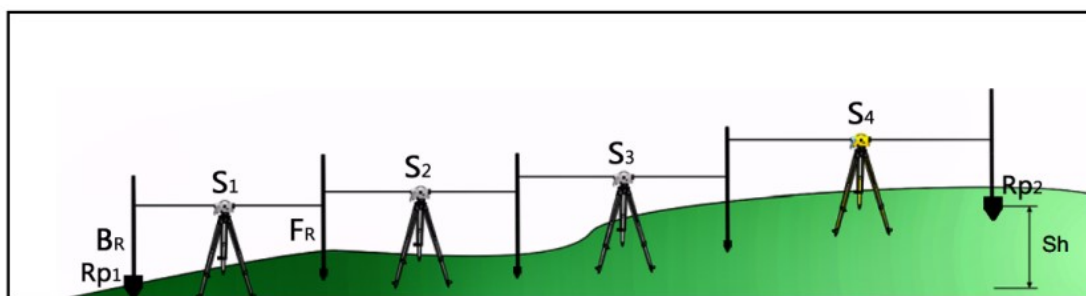
2.18-rasm. Nivelir yo'li
