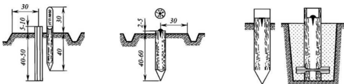
2.5-rasm. S'yomka tarmoqlarini nuqtalarini vaqtincha mahkamlash belgilari
