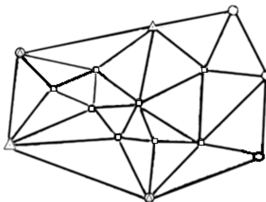
2.1-rasm. Tarmoq qurish usulida s'yomka asosini rivojlantirish sxemasi:
