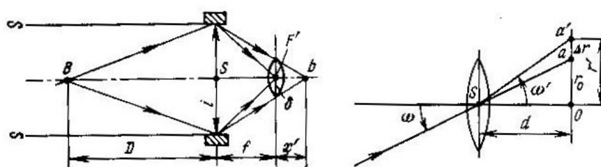
4.5-rasm. Ko'rish maydoni va distorsiya vujudga kelishi
