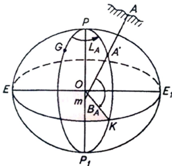
1.7-rasm. Geodezik koordinatalar sistemasi
