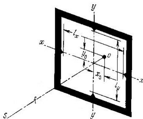
4.17-rasm. Aerofotosuratning ichki orientirlash elementlari
