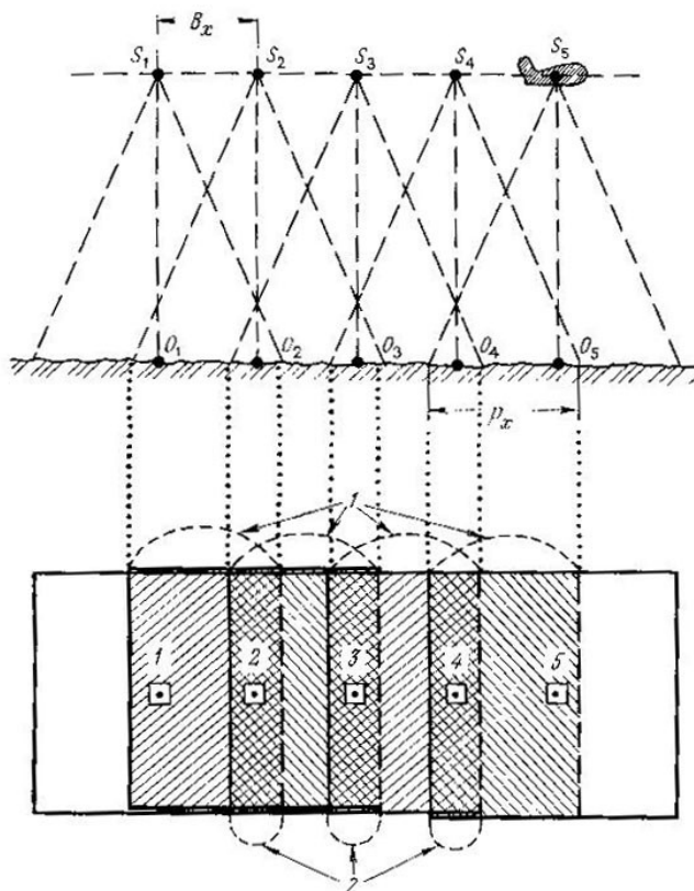
4.8-rasm. Bitta marshrutli aerofotosʻyomka va suratga olish bazisi
