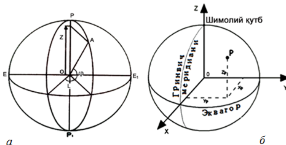
1.5-rasm. Geotsentrik koordinatalar sistemasi:
