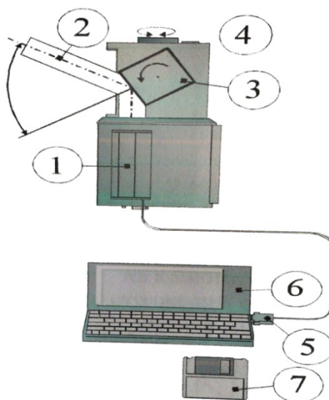
2.22-rasm. Er usti lazer skanerlash sistemasi:
