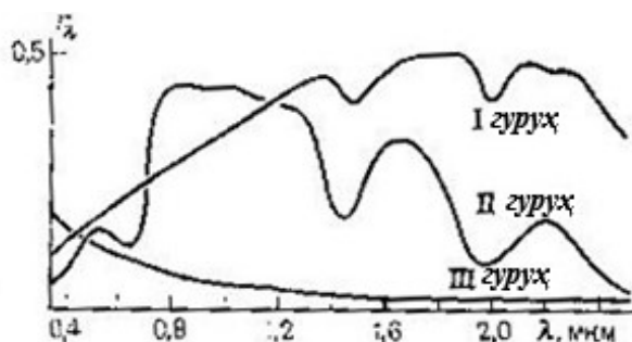
4.4-rasm. Tabiiy ob'ektlarning spektr yorug'lik koeffitsienti
