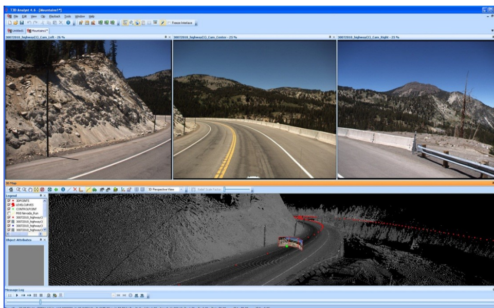
3.13-rasm. Trident Analyst yordamida ishlab chiqilgan mobil fotos'yomka va lazer skanerlash natijalari
