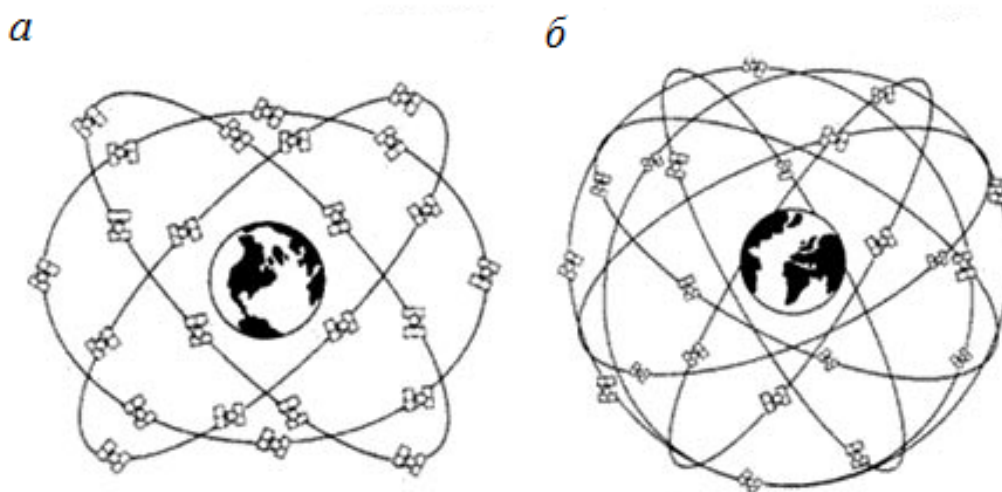
3.5-rasm. Sun'iy yo'ldoshlarning orbital guruhlari sxemasi: a– GLONASS sistemasida; b– GPS sistemasida
