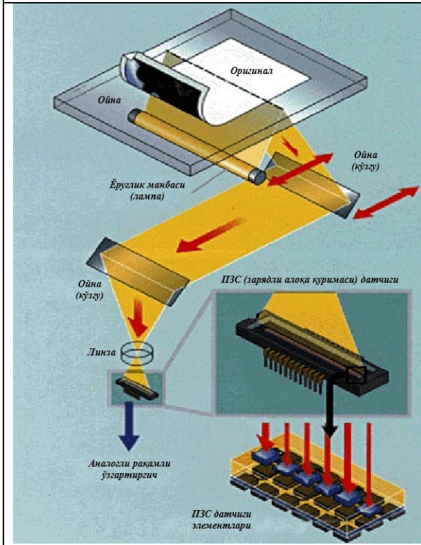
5.1-rasm. Плanshetli skaner va uning ishlash sxemasi
