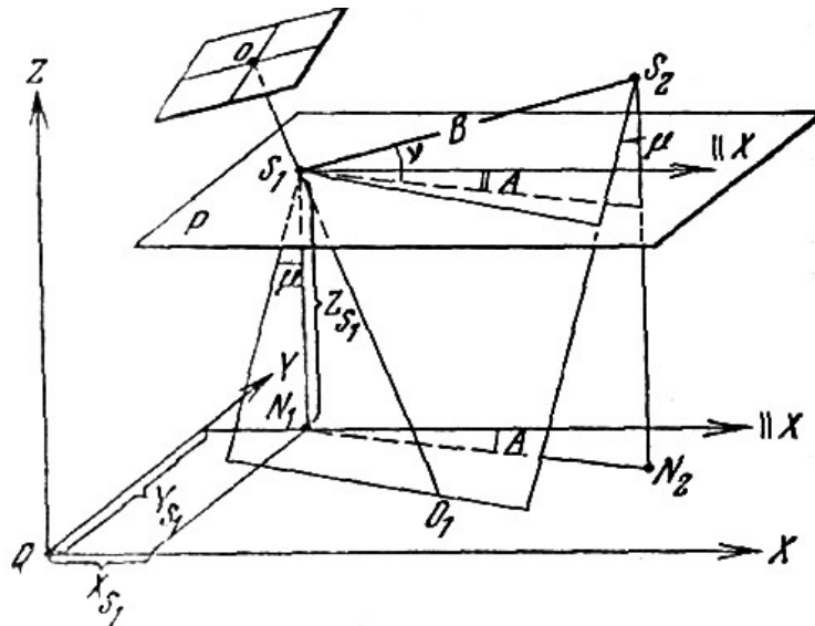
4.22-rasm. Tashqi orientirlash elementlari
